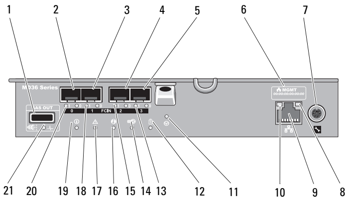
图 3-1. MD3600f 系列光纤信道 RAID 控制器模块
